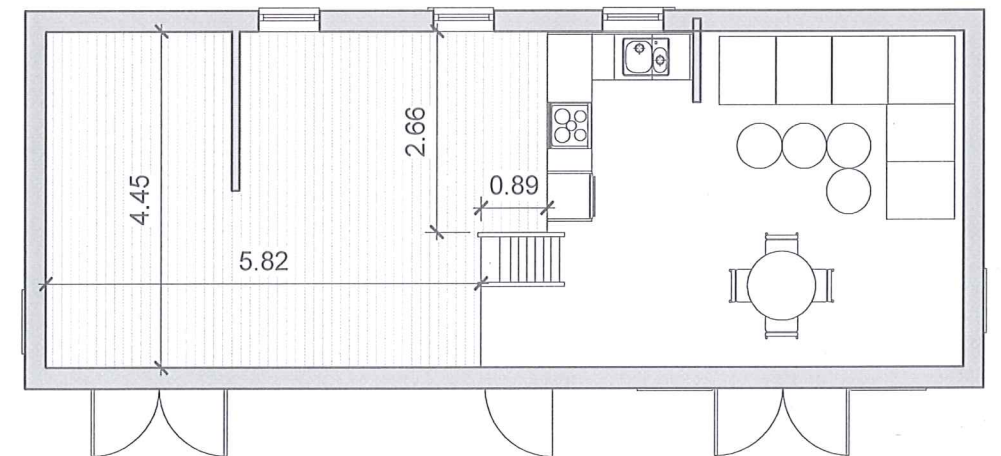
2 PLAN 2 1 : 100
